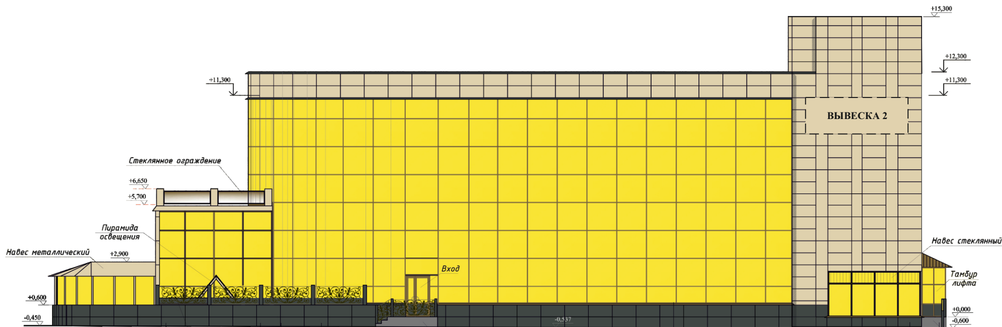
ЧЕРТЕЖ ФАСАДА ВИД 2.
